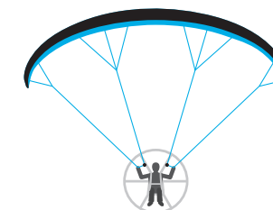
Schema 3 Das Herunterziehen der Bremsen auf gewohnte Art und Weise wird beides, nämlich das TST und die Bremsen ansprechen
